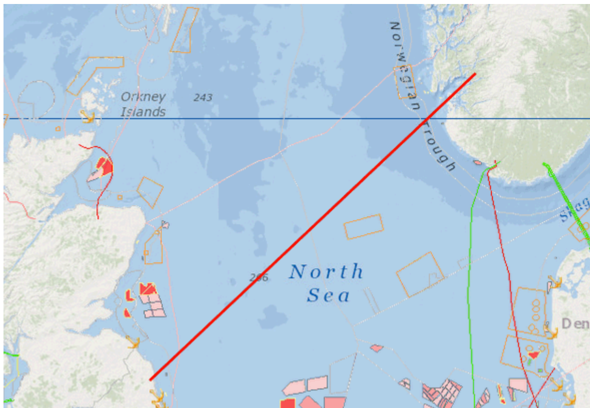
Der NSN Link wird die längste Gleichstromverbindung. Die 720 Kilometer lange Seekabelverbindung verläuft zwischen dem englischen Blyth und dem norwegischen Kvilldal.
