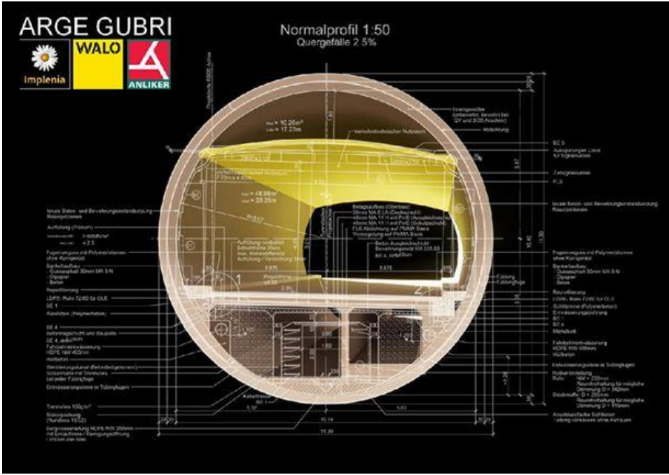
Visualisation BIM de la rénovation des tubes existants du tunnel du Gubrist (image : ©Consortium GUBRI).
